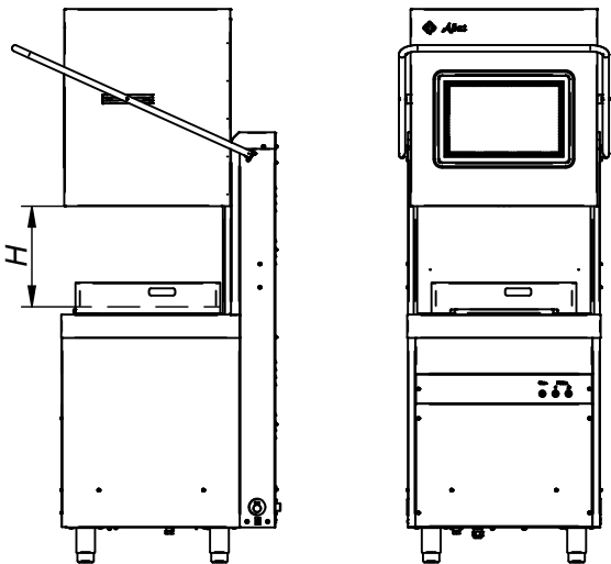
Рис. 4. Высота проема моечной камеры Н машин купольного типа, на примере машины МПК-700К
